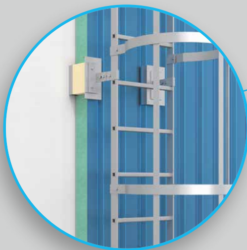
TRAPEZOIDAL SHEETMETAL THERMAL PANEL
